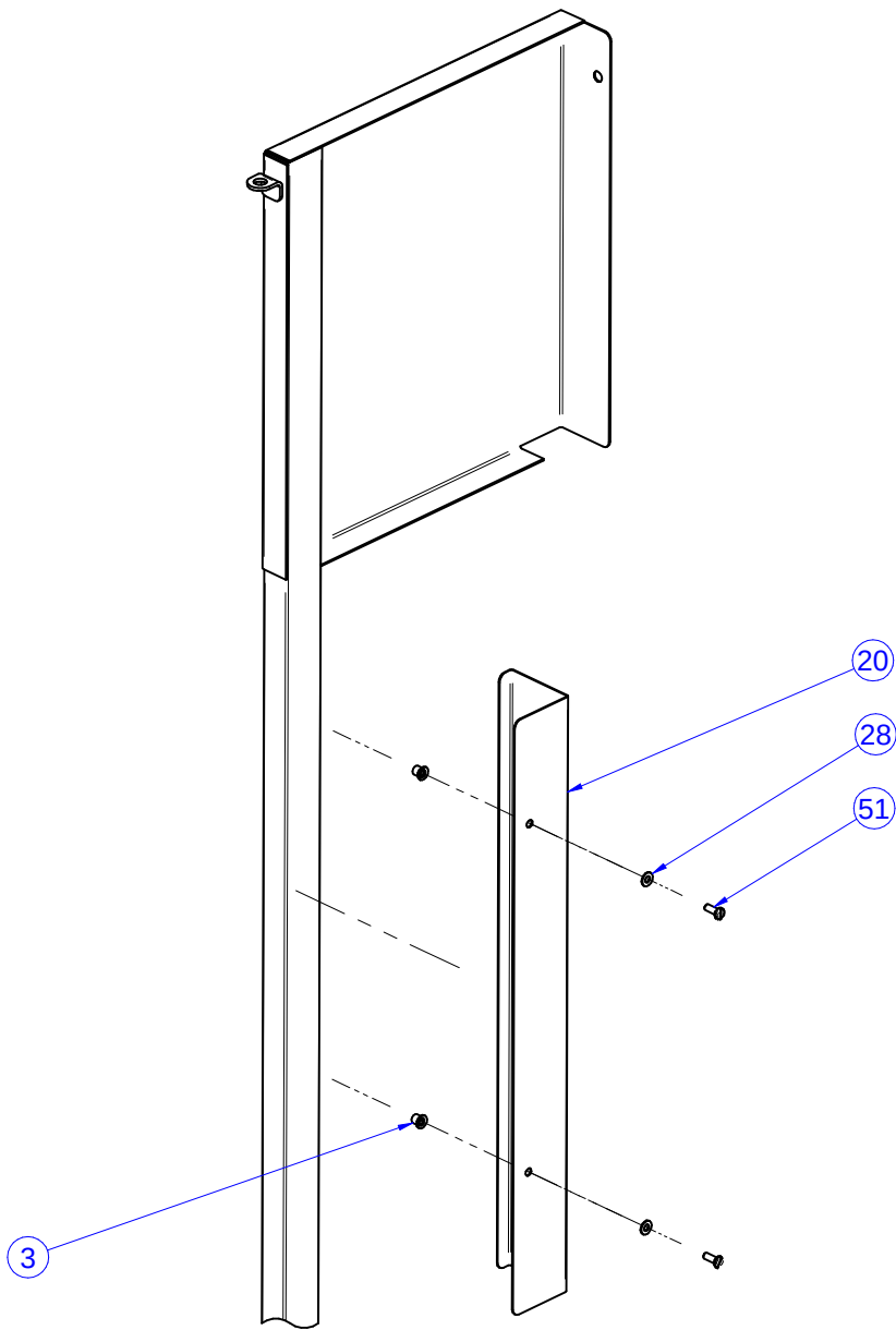
MONTAGEM DO GUIA DA LÂMINA, TACO DO GUIA DA LÂMINA E PROTETOR DA LÂMINA
