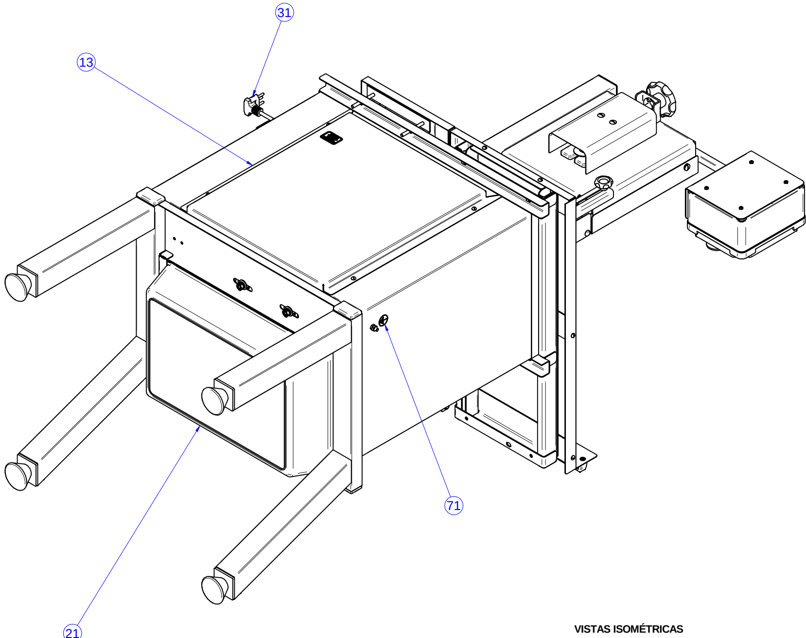
VISTAS ISOMÉTRICAS
