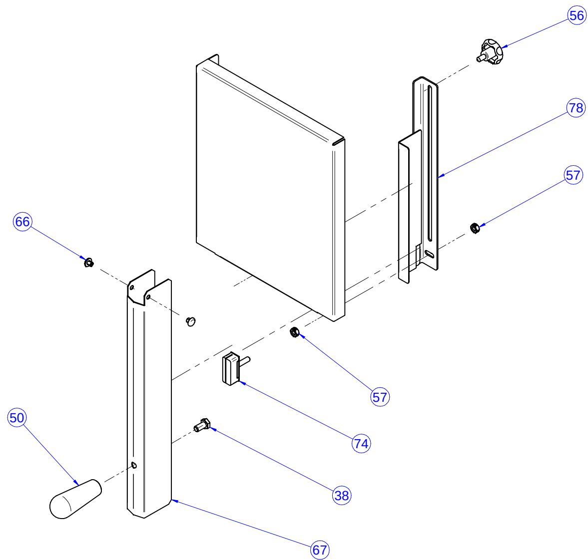
MONTAGEM DO GUIA DA LÂMINA, TACO DO GUIA DA LÂMINA E PROTETOR DA LÂMINA
