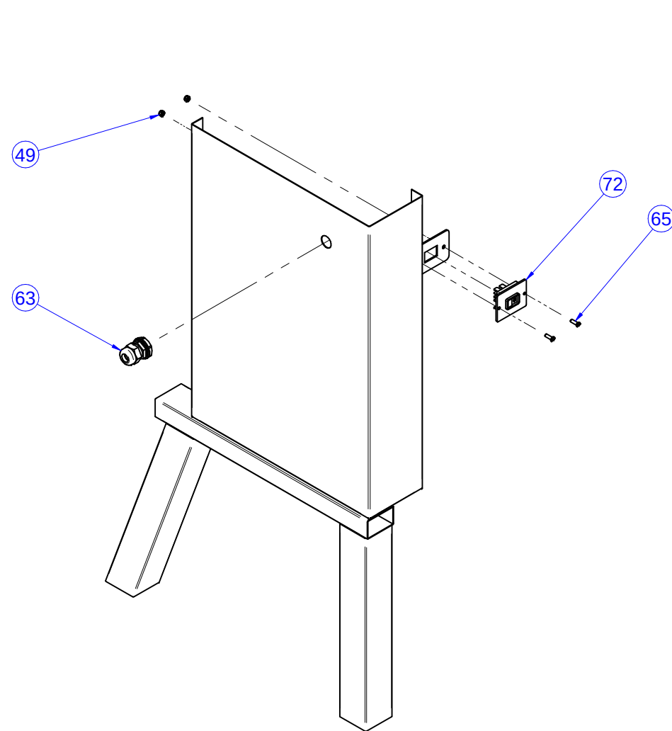
MONTAGEM DA CHAVE BIVOLT, E PRENSA CABO
