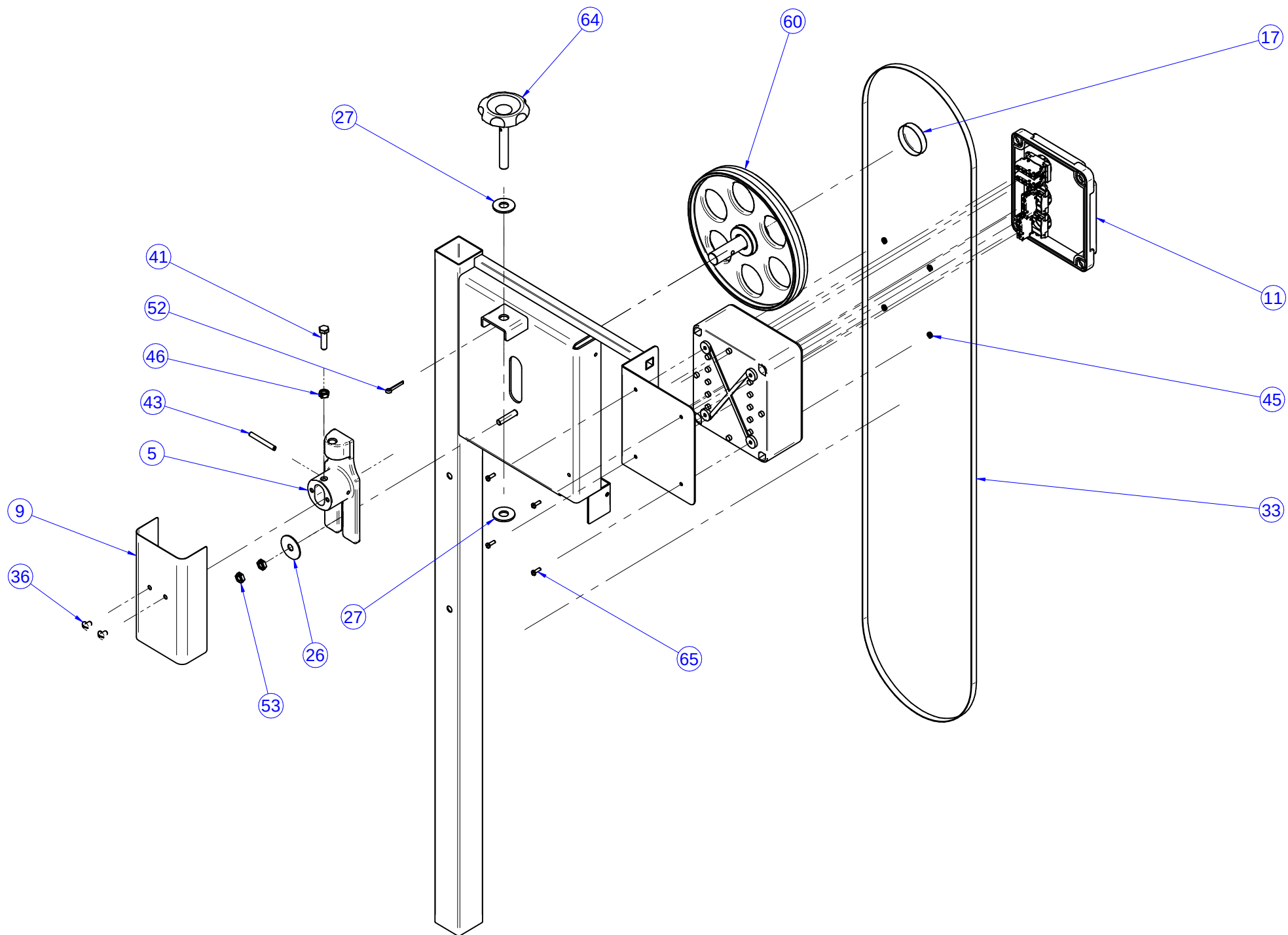
MONTAGEM DO VOLANTE SUPERIOR, ESTICADOR DA SERRA, SERRA E CAIXA COMPONENTE ELÉTRICO
