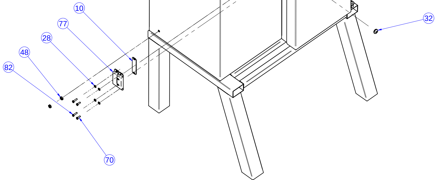
MONTAGEM DO SENSOR DE SEGURANÇA RIOCON, PARAF. E PORCAS P/ FIXAR FIO TERRA E PASSA FIO
