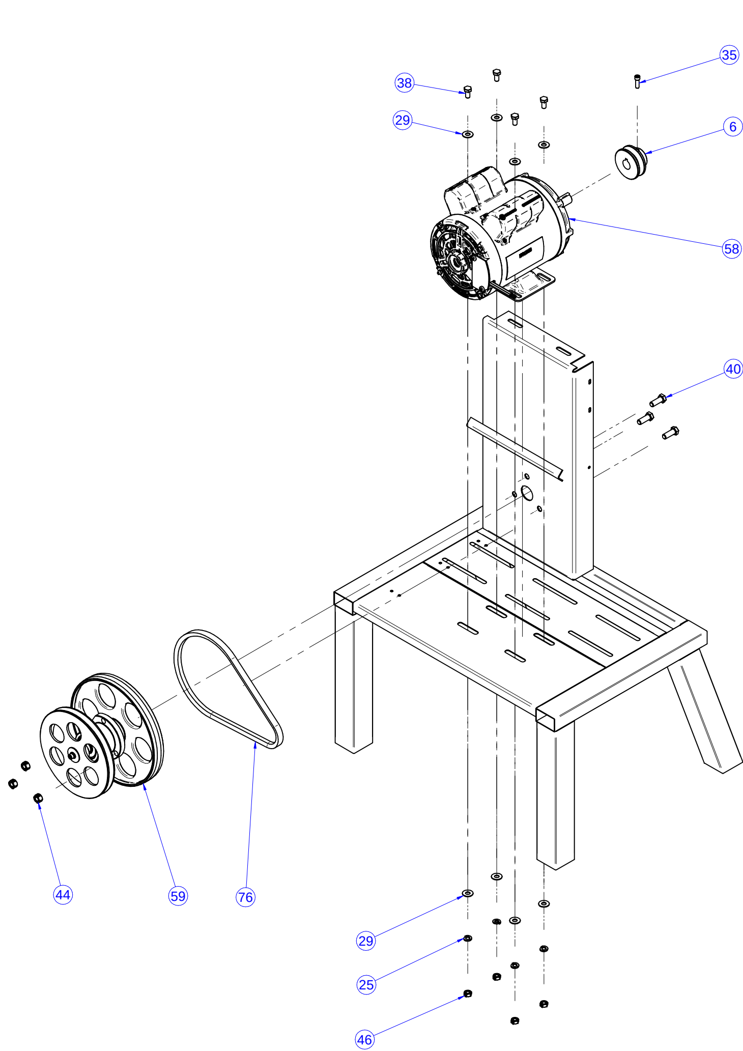
MONTAGEM MOTOR E MANCAL
