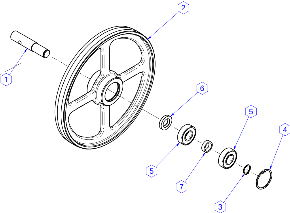
VOLANTE COMPLETO (SUPERIOR)
