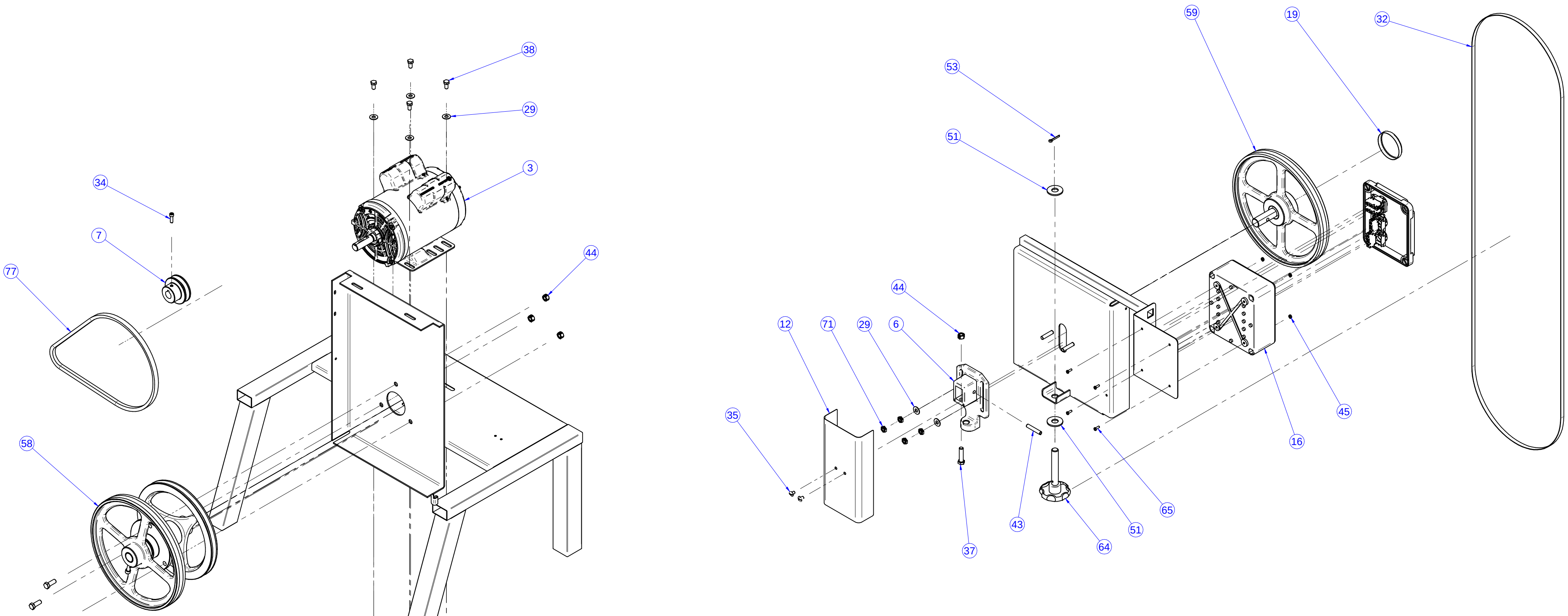
MONTAGEM ESTICADOR DA SERRA, SERRA, VOLANTE SUPERIOR E CAIXA COMPONENTES ELÉTRICOS
